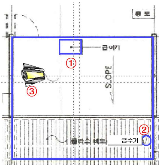
<그림 1> 부분 슬랏돈사 돈방 평면도
