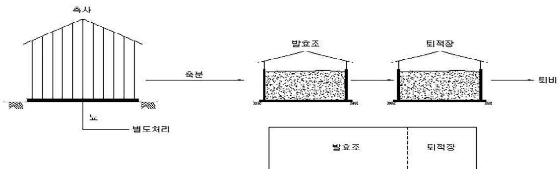
퇴비사의 처리공정도
